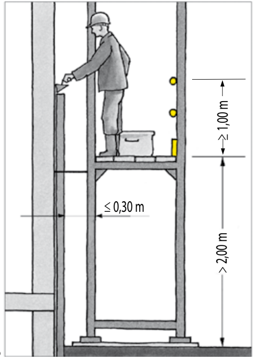
36 Schnittdarstellung – auch die Seiten sind zu sichern.
